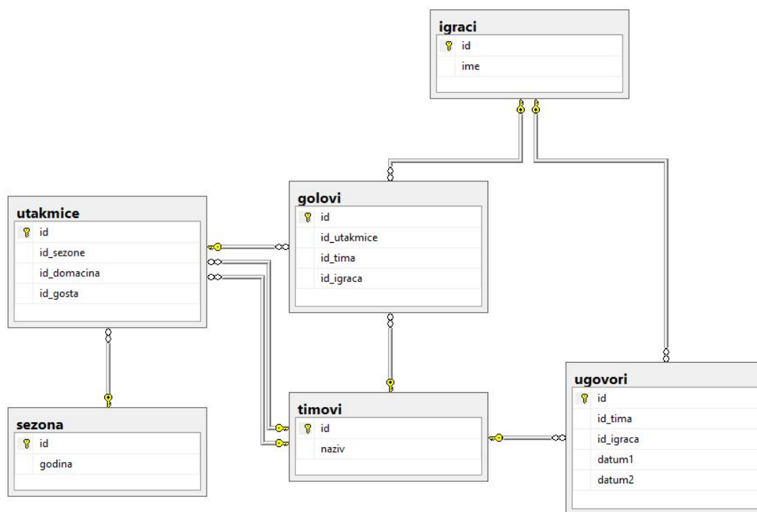
Слика 1: Модел базе података
