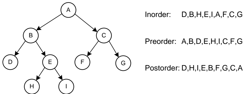
Slika ### Redosled obilaska binarnog stabla
