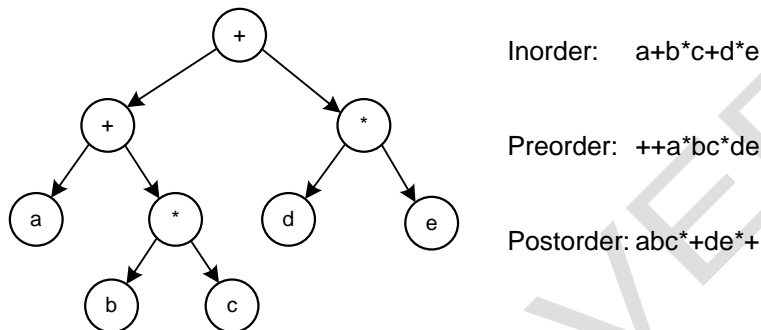
Slika ### Aritmetički izraz predstavljen binarnim stablom
