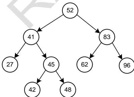
Slika ### Binarno stablo za pretraživanje
