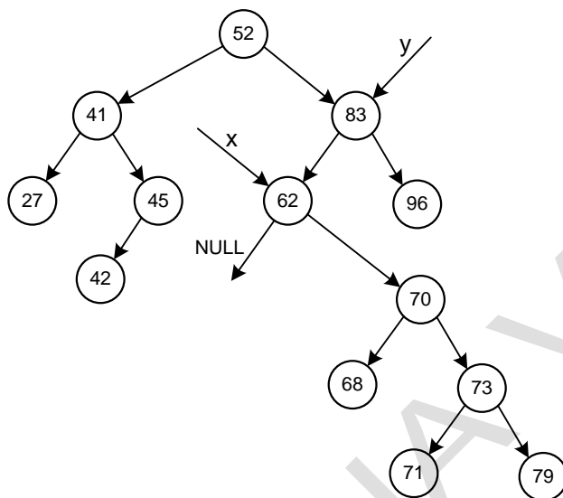
Slika ### Binarno stablo pre brisanja čvora na koji pokazuje x
